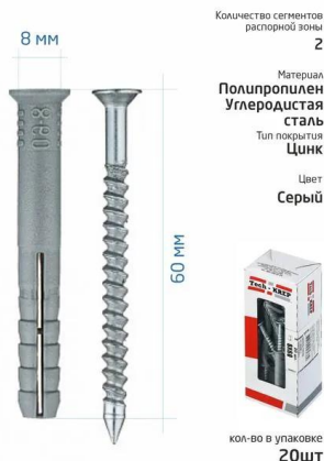
Дюбель-гвоздь SM-L 8х60 потайная манжета
