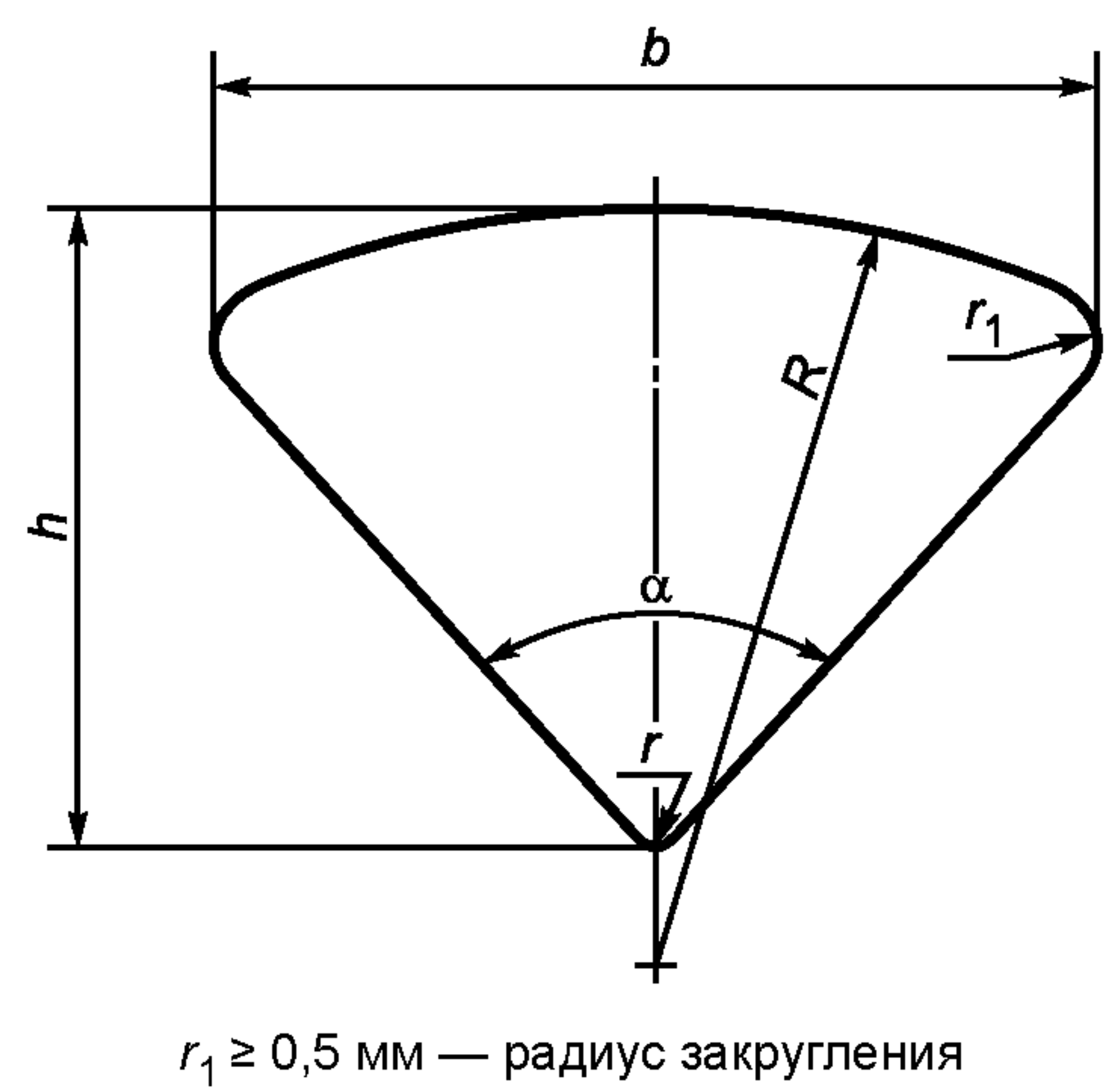
Рисунок А.2 — Конструкция секторных однопроволочных алюминиевых жил
